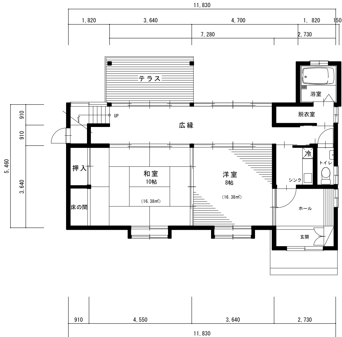
1階平面図
