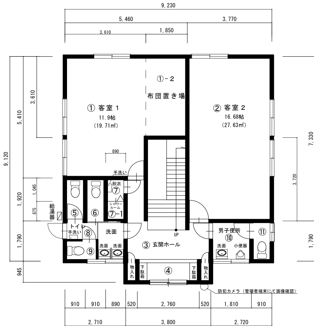
1階平面図
